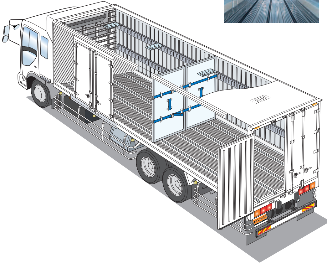
移動軟質脱着式
