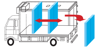
B 移動両吊り式
