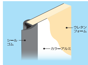
デッキパネル 硬質ウレタン心材の扉で非常に軽いのが特徴です。
