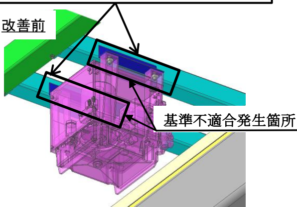
ウイングパワーユニット取付ブラケット
